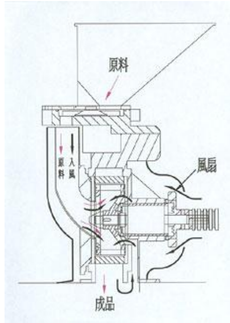
氣流循環特別設計構造
